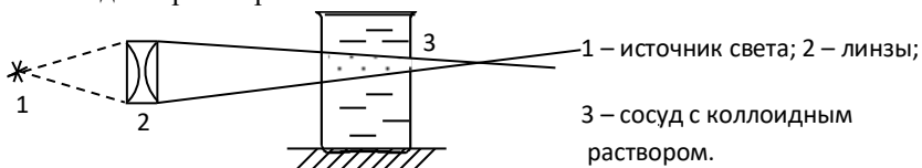
Рисунок 1 – Схема эффекта Тиндаля
