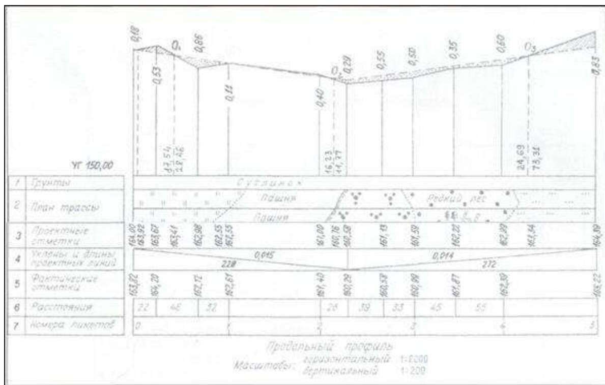
Рис.18. Продольный профиль трассы
