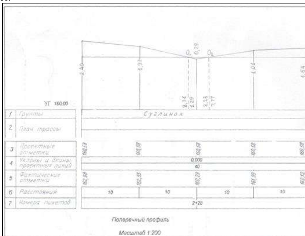
Рис.20. Поперечный профиль трассы РАБОТА С КАРТОЙ
