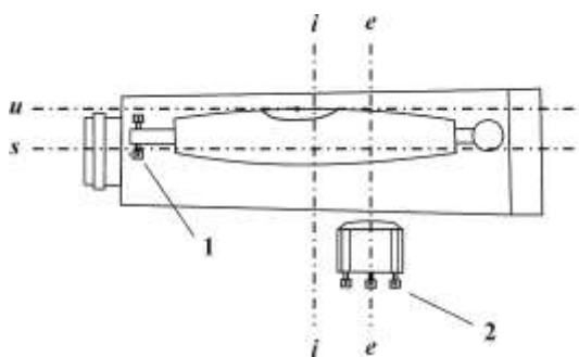
Рисунок 18. Оси и исправительные винты нивелира: ss – визирная ось зрительной трубы; ii – ось вращения прибора; uu – ось цилиндрического уровня; ee – ось круглого уровня; 1 – исправительные винты цилиндрического уровня; 2 – исправительные винты круглого уровня.
