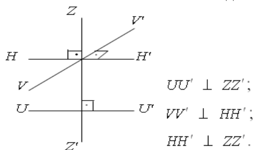
Рисунок 7. Схематическое расположение основных осей теодолита
