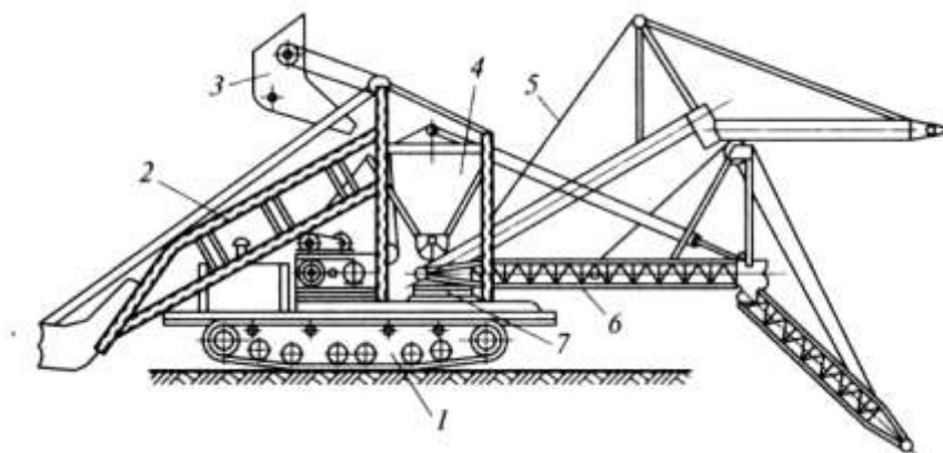
Рисунок 3. Самоходный бетоноукладчик.
