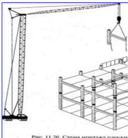
Рисунок. Схема монтажа плоских Н – образных рам.
