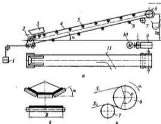
Рисунок 1. Ленточный конвейер
