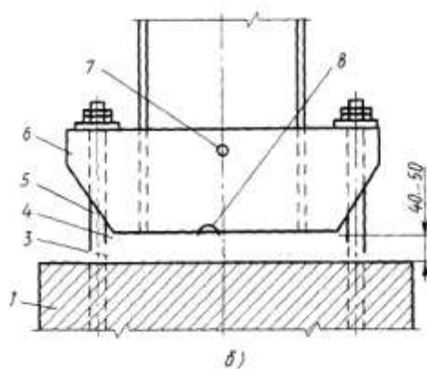
Рисунок 2.1 Схемы установки стальных колонн на фундаменты: б — на заранее установленные плиты; / — фундамент, 2 — подкладки, 3 — подливка из раствора, 4 — опорная плита, 5 — анкерные болты, 6 — опорная база колонны, 7 — строповочное отверстие, 8 — отверстие для удаления воды
