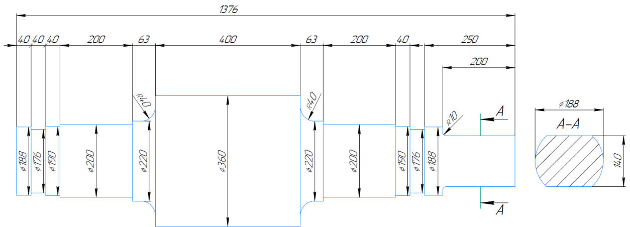
Рис. 1. Основные размеры рабочего валка
