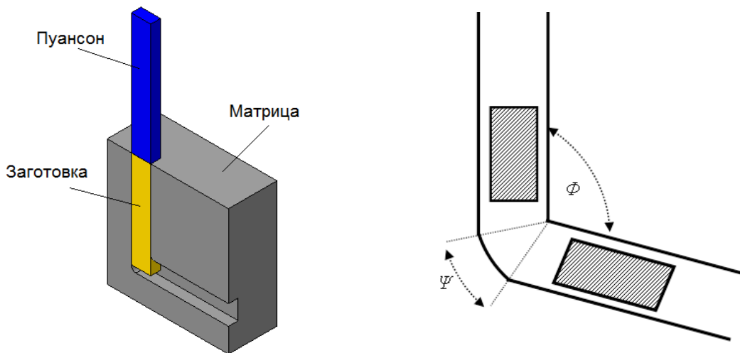
Рис. 1. Схема процесса РКУП
