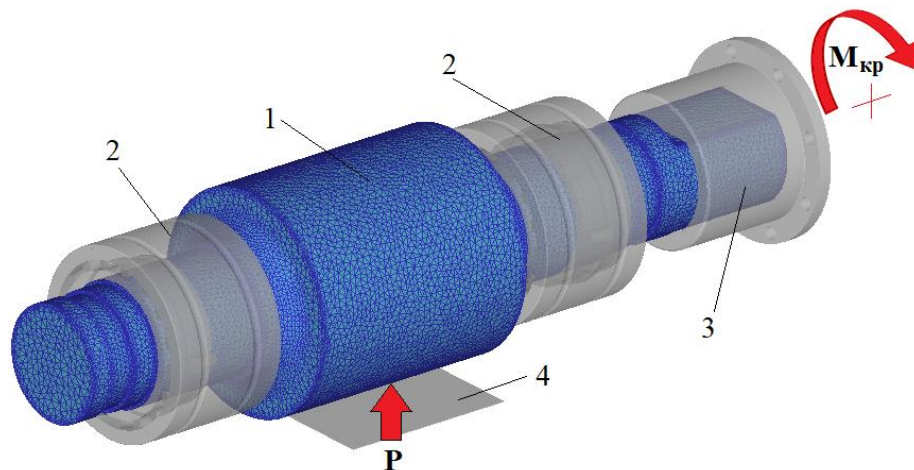
Рис. 4. САЕ-модель: 1 – рабочий валок; 2 – подшипники; 3 – полумуфта; 4 – прокатываемый лист (полоса)
