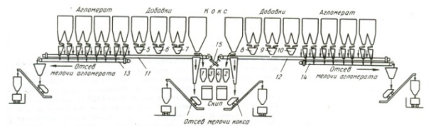
Рис. 5. Система шихтоподачи доменной печи объемом 2000 м 3 КМЗ (1962 г.)
