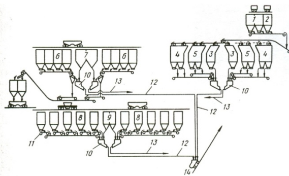
Рис. 6. Схема шихтоподачи доменной печи "Atapanda" объемом 2032 м 3 : 1 – бункера окатышей; 2, 3 – бункера известняка; 4 – бункера агломерата и руды; 5 – бункера окатышей и руды; 6, 7 – бункера кокса; 8 – бункера добавок; 9 – бункер скрапа; 10 – весовые воронки; 11–13 – ленточные весы; 14 – скип
