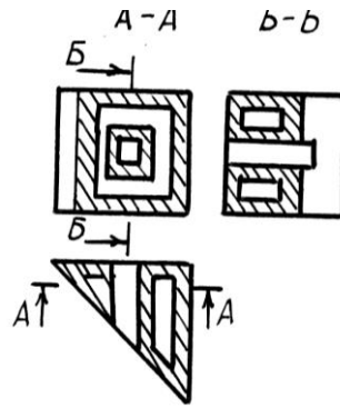
Рис. 2.3 Неразъемная оболочка по контуру детали
