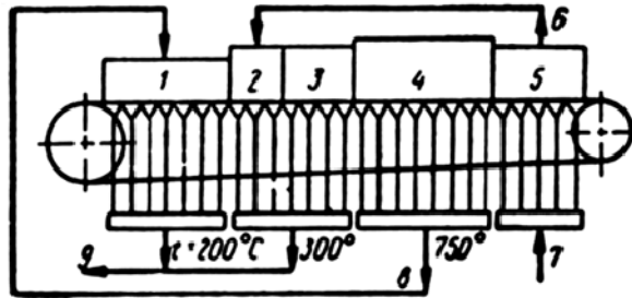
Схема обжига окатышей на конвейерной обжиговой машине
