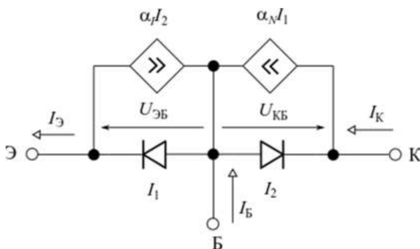
Рисунок 4.2 – Модель Эберса-Молла для pnp -транзистора
