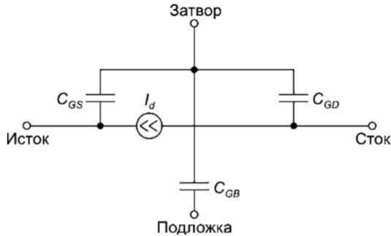
Рис. 5.1 – Емкостная модель Мейера
