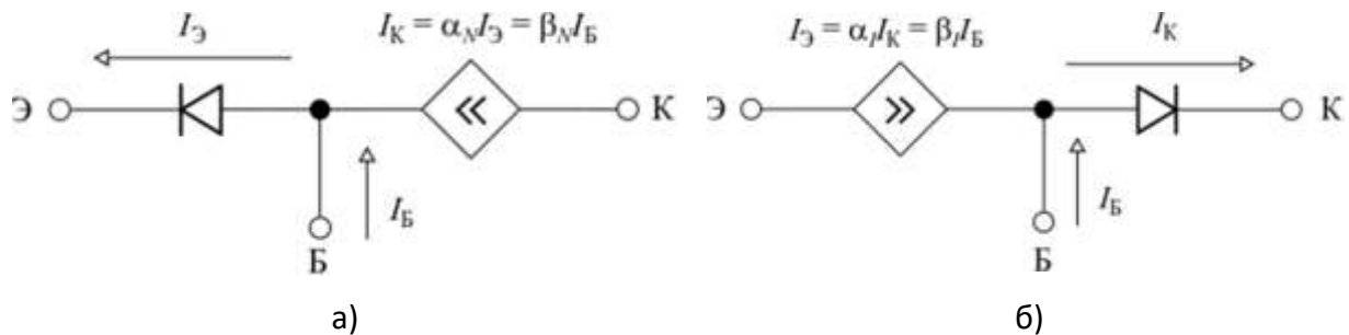
Рисунок 4.3 – Упрощённые схемы модели Эберса-Молла для npn -транзистора:
