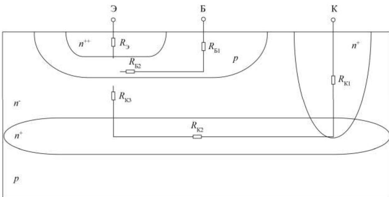
Рисунок 4.7 – Структура интегрального биполярного npn -транзистора с сопротивлениями квазинейтральных областей
