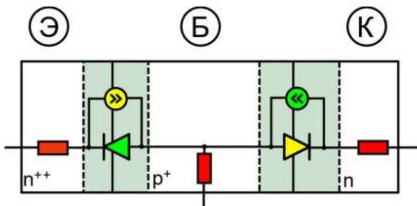
Рисунок 4.1 – Структура pnp -транзистора для формирования модели Эберса-Молла
