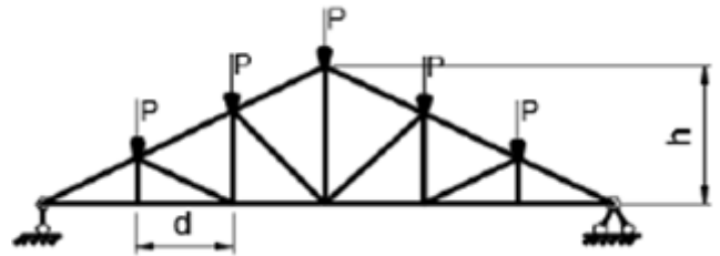
Рисунок 1 – Расчетная схема фермы
