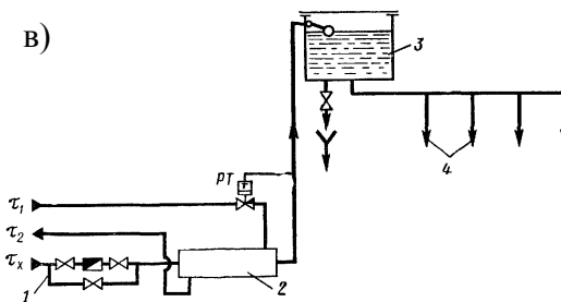
1 — водопроводная вода; 2 — секционный водонагреватель; 3 — верхний бак-аккумулятор с поплавковым краном; 4 — к водоразборным приборам; РТ — регулятор температуры
