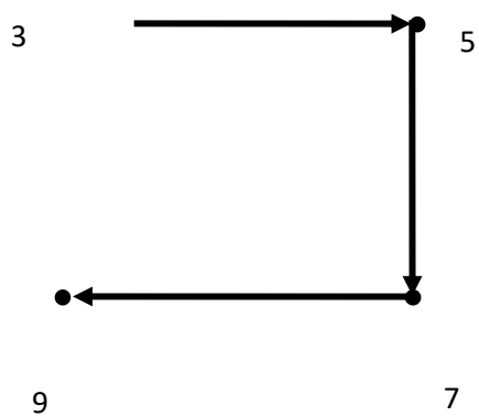
Рис.7 Граф отношения Р.
