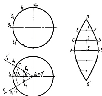
Рисунок 17. Развертка сферы с 6 сегментами
