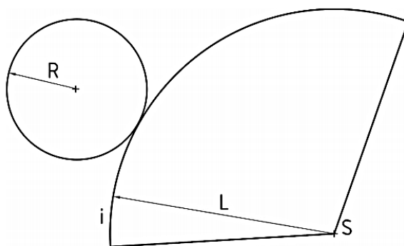
Рисунок 14. Развертка конуса
