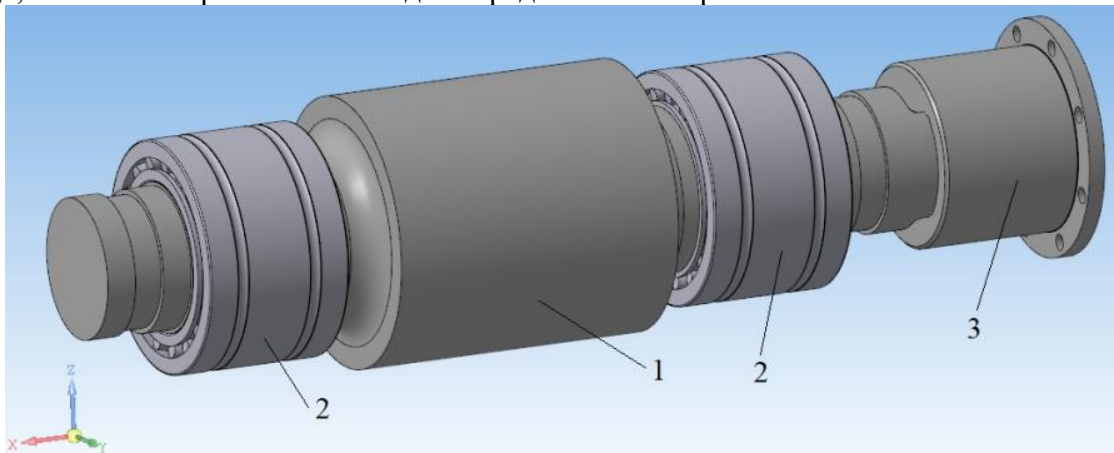
Рис. 3. CAD-модель сборки: 1 – рабочий валок; 2 – подшипники; 3 – полумуфта
