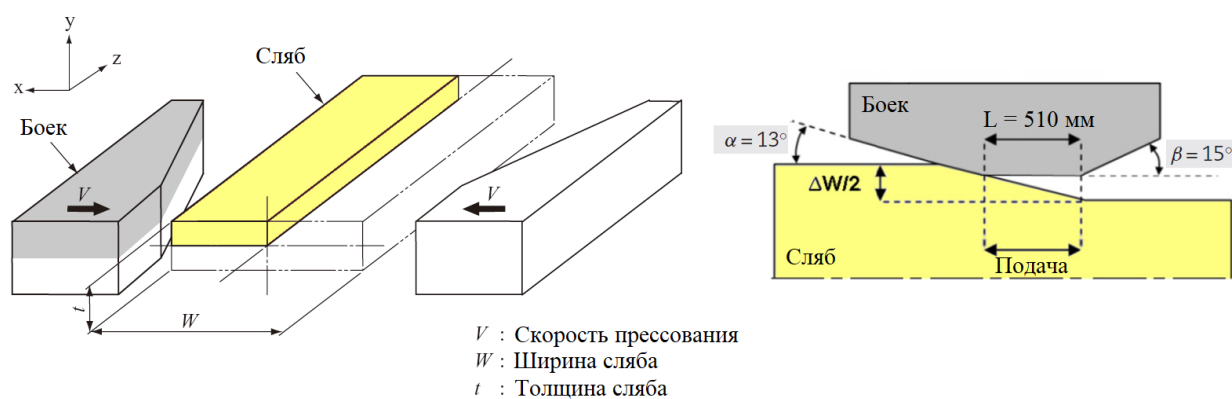
Рисунок 2 – Схема редуцирования слэба прессом
