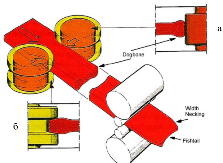
Рисунок 1 – Схема деформации слэбов по ширине: а – гладкими вертикальными валками (эджерами); б – калиброванными вертикальными валками (эджерами)
