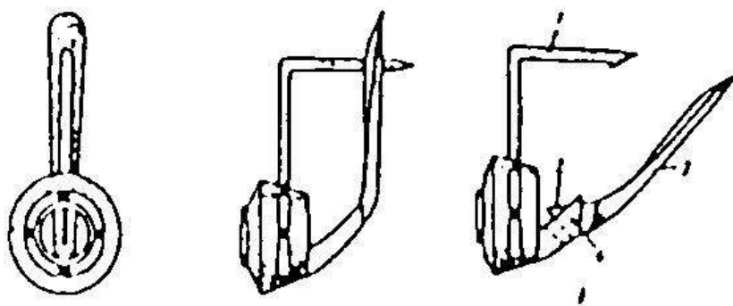
а - закрытое положение замка; б - открытое положение замка; 1 - пружинный крючок; 2 - флажок; 3 - швенза
