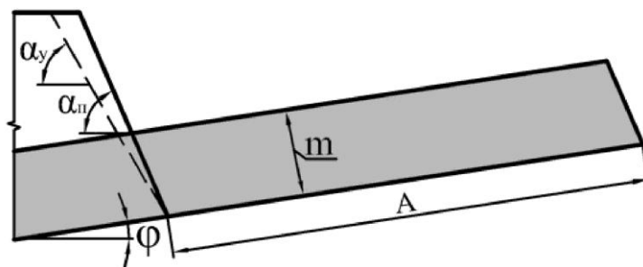
Рис. 3.1 – Параметры заходки по угольному пласту: m – мощность пласта, м; A – ширина заходки, м; \alpha_y ,
