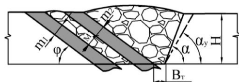
Рис. 5.1 – Параметры залегания пластов на уступе, разрабатываемых по схеме с проходкой разрезной траншеи со стороны кровли верхнего пласта: Н – высота вскрышного уступа, м; φ – угол залегания пластов, град; m_1 и m_2 – соответственно мощность нижнего и верхнего пласта свиты, м; М – мощность между-пластья, м; B_T – ширина разрезной траншеи по дну ( B_T = 3\text{ м} ); \alpha_y , α – соответственно устойчивый и рабочий углы откоса вскрышного уступа, град
