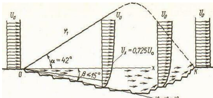
Рециркуляционная схема:
