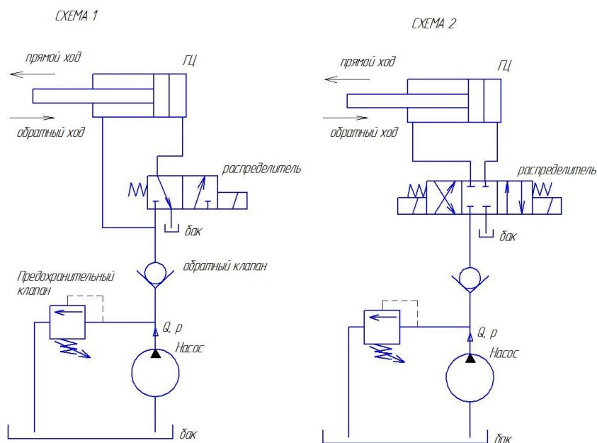
Рисунок 1 – Гидравлические схемы подключения гидроцилиндра
