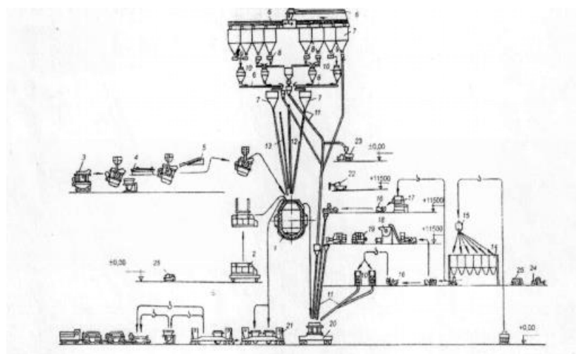
Рисунок 1. Технологическая схема работы конвертерного цеха: 1-конвейер; 2-совок с ломом; 3-чугуновозный ковш; 4-машина для скачивания шлака; 5-устройство для
