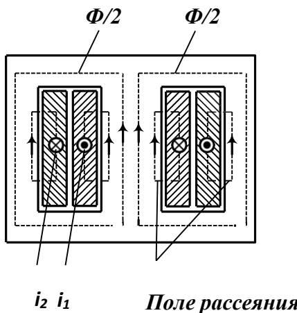
Рис. 2. Магнитное поле трансформатора
