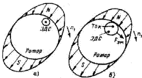
Рис. 10. Проводник ротора во вращающемся магнитном поле статора: а - наведение ЭДС в проводнике ротора; б - возникновение электромагнитных сил
