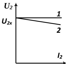
Рис. 6. Внешние характеристики идеализированного (1) и реального (2) трансформаторов
