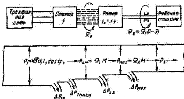
Рис. 11. Диаграмма преобразования энергии в асинхронном двигателе
