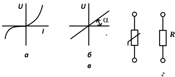
Рис. 3. Нелинейная (а) и линейная (б) ВАХ приемников, условные обозначения нелинейного (в) и линейного (г) резистивных элементов
