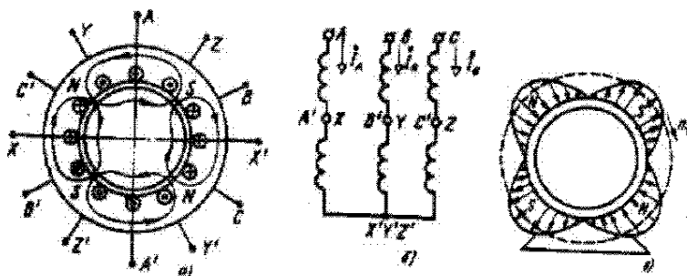
Рис. 9. Эпюра вращающегося магнитного поля: а - распределение тока по проводникам обмотки статора; б - схема соединения катушек обмотки статора; в — эпюра магнитного поля двухполосной машины
