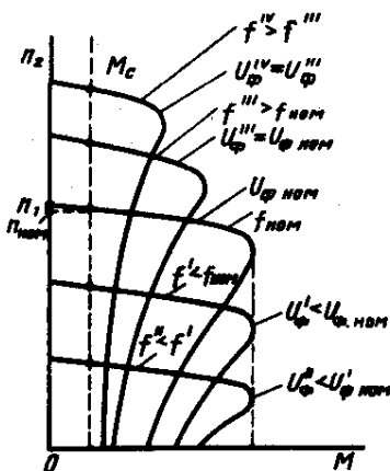
Рис. 16. Механические характеристики двигателя с частотным регулированием скорости
