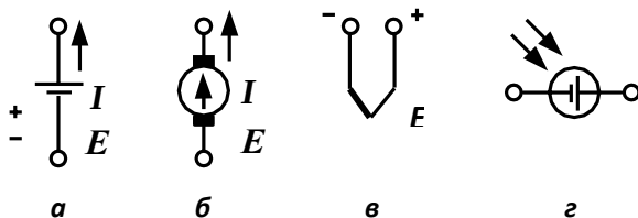
Рис. 1. Обозначения источников постоянного тока на схемах: a – гальванический элемент и аккумулятор; b – генератор постоянного тока; в – термопара; г – фотоэлемент
