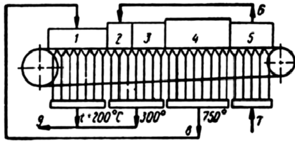
Схема обжига окатышей на конвейерной обжиговой машине
