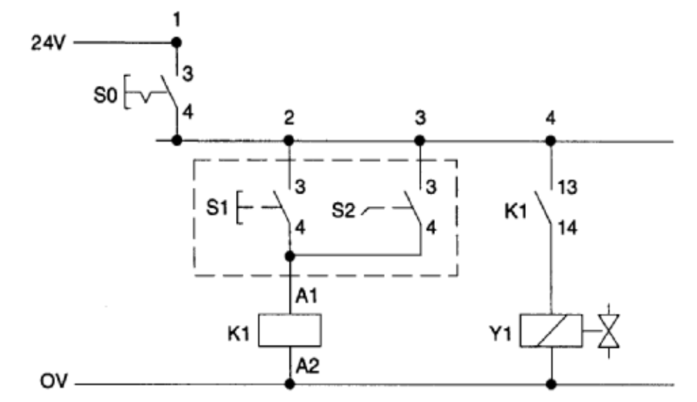
2 электрическая схема
