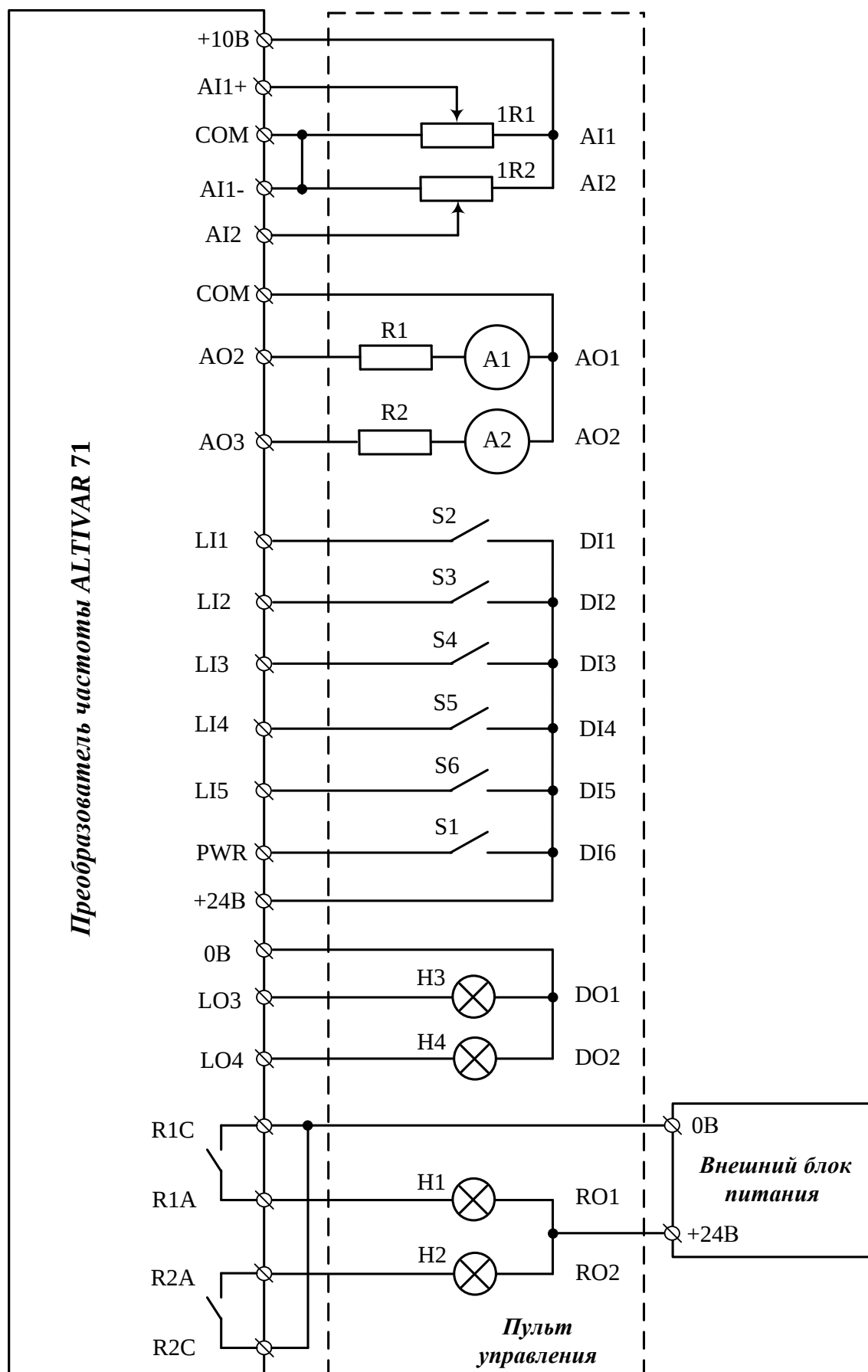
Рисунок 3. Схема подключения пульта управления к ПЧ ALTIVAR 71
