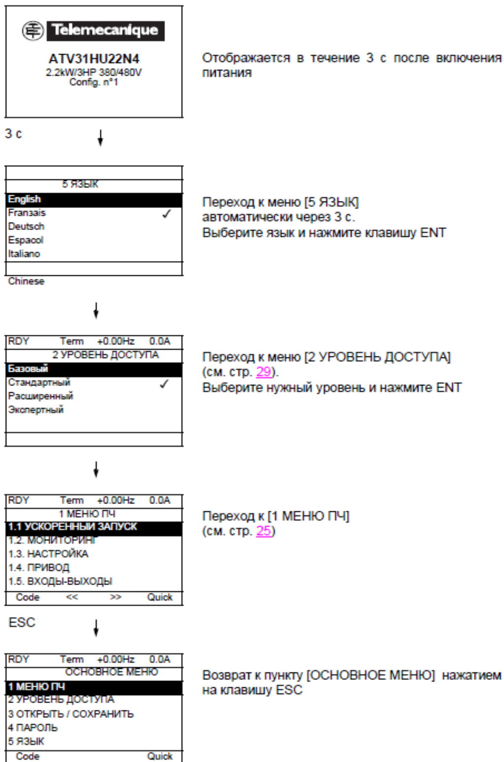
Рисунок 4. Графический терминал. Первое включение ПЧ
