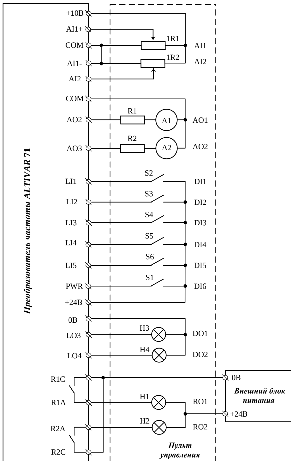
Рисунок 3. Схема подключения пульта управления к ПЧ ALTIVAR 71
