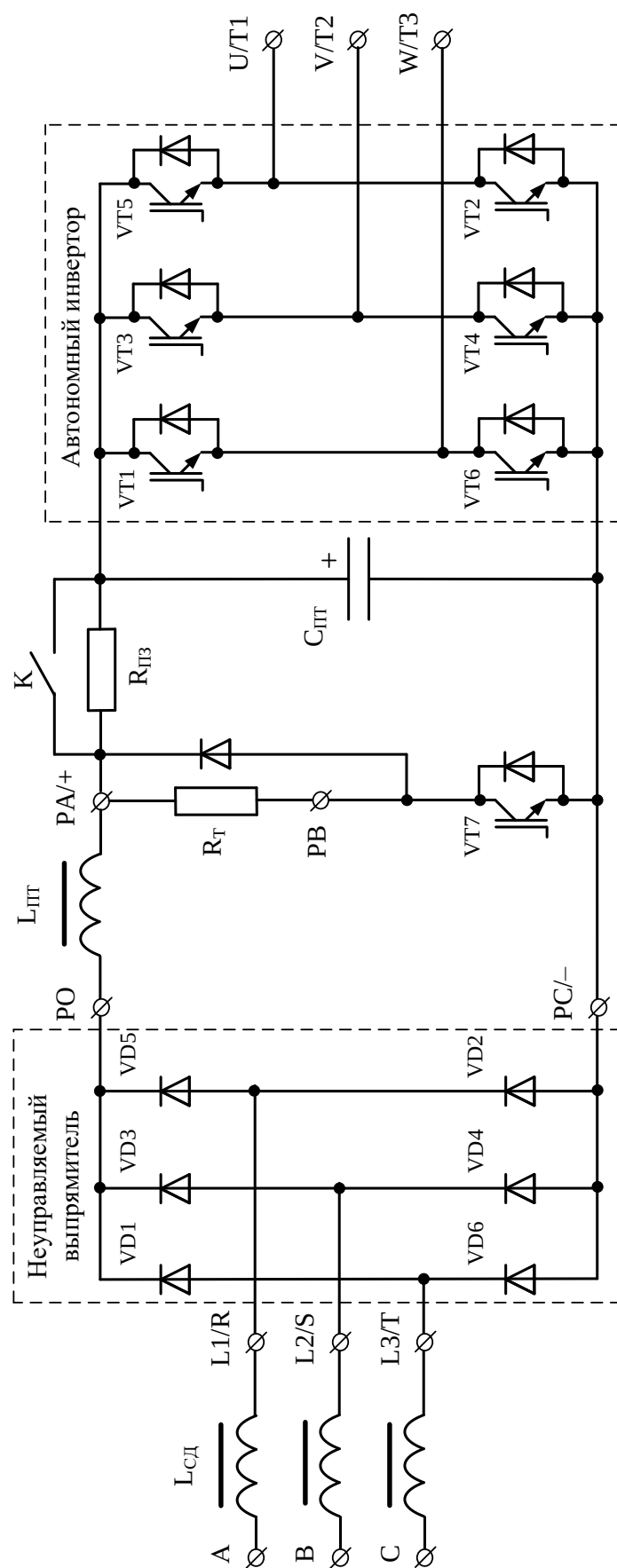
Рисунок 2. Силовые цепи преобразователя частоты ALTIVAR 71
