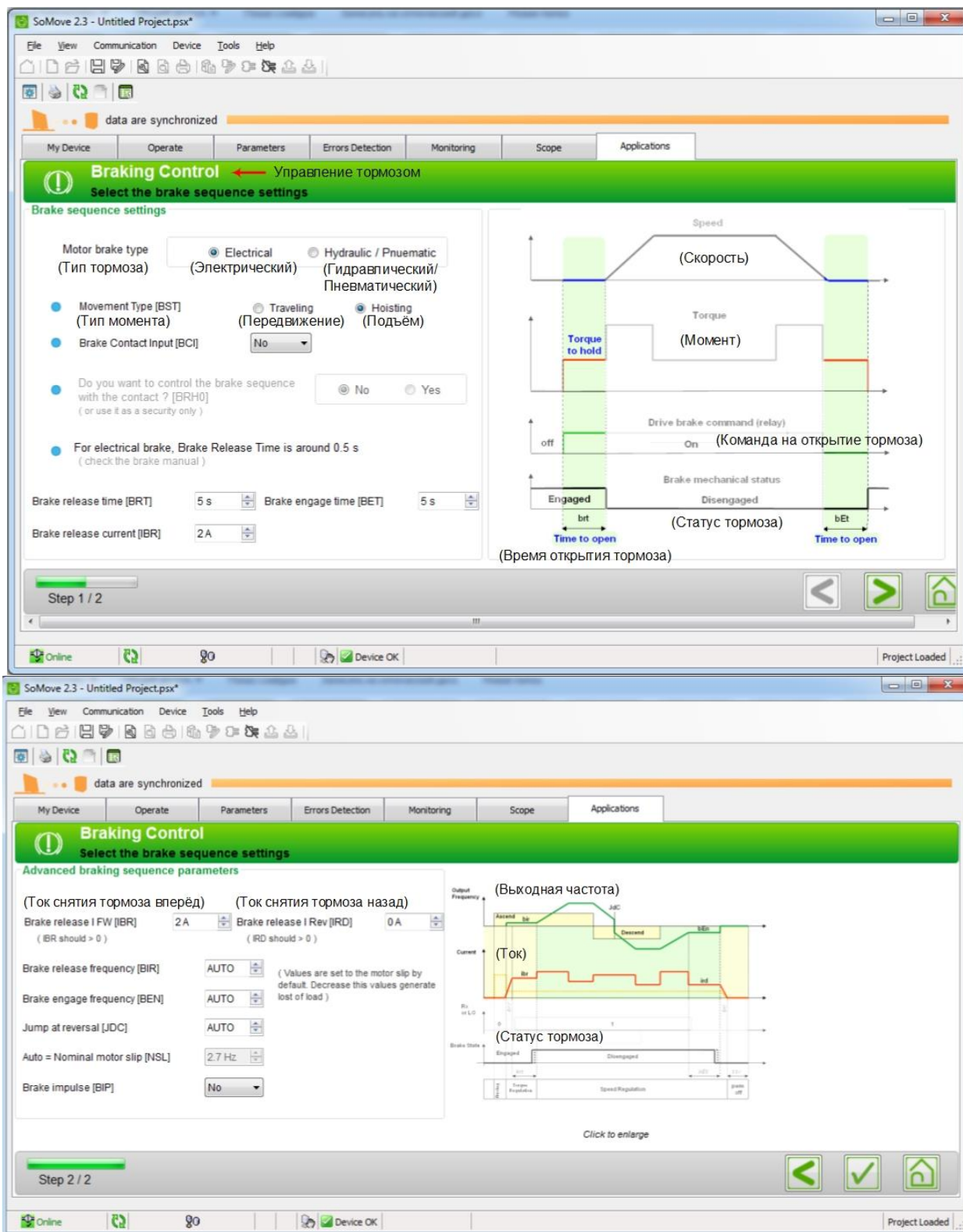
Рисунок 17 – Управление стояночным тормозом
