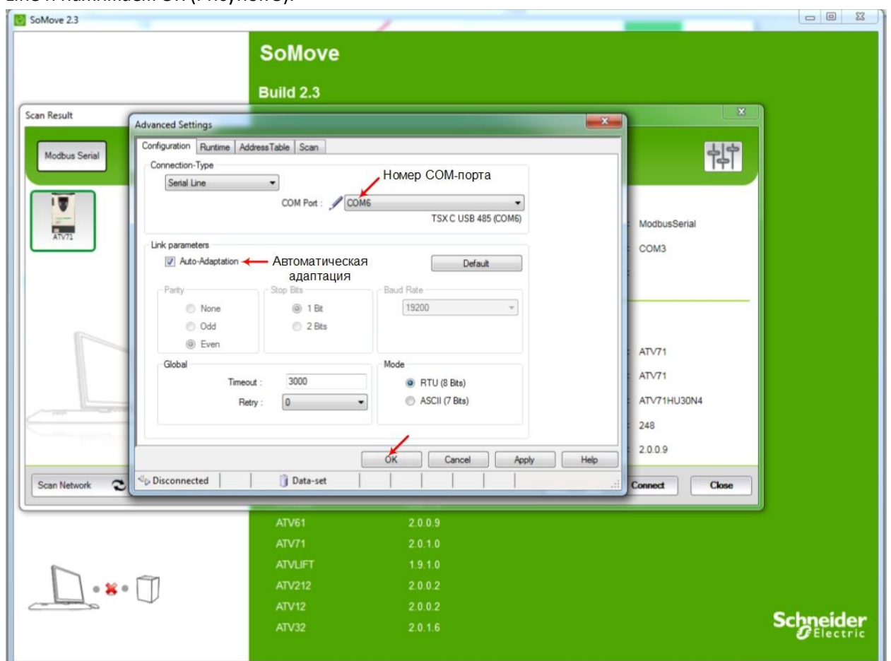
Рисунок 5 – Настройки соединения
