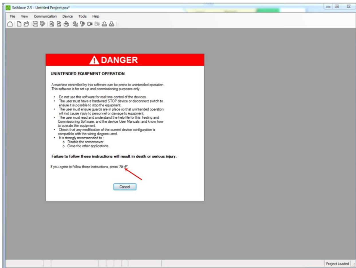
Рисунок 8 – Подтверждение подключения
