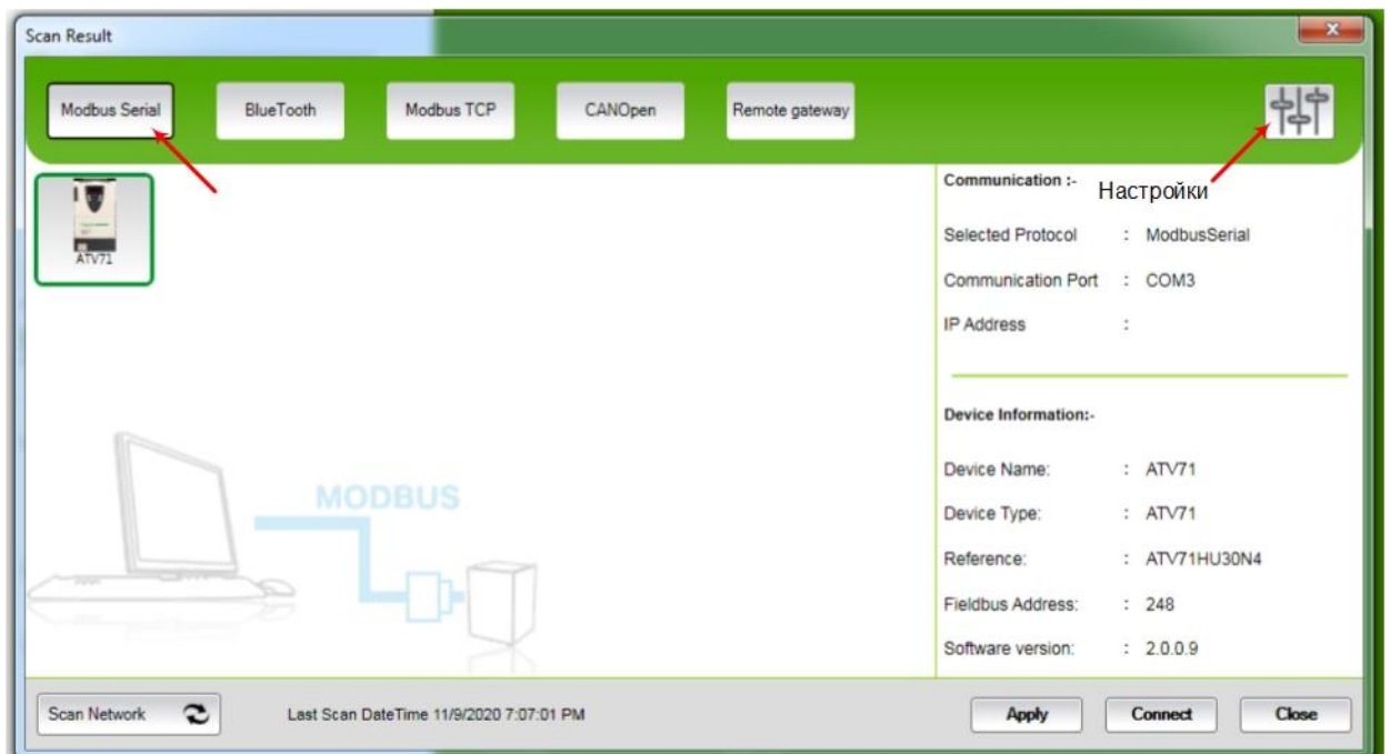
Рисунок 4 – Найденные устройства
