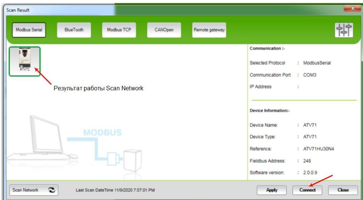
Рисунок 6 – Найденные устройства
