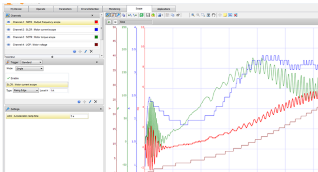
Рисунок 15 – Осциллограммы пуска двигателя
