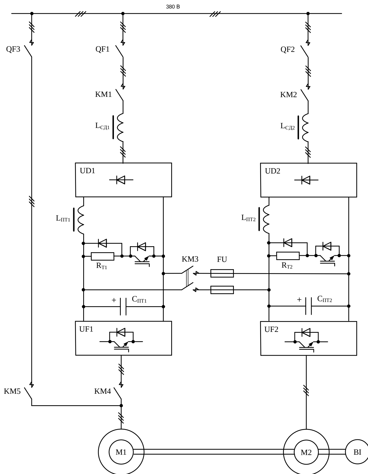
Рисунок 1. Однолинейная схема лабораторного стенда
