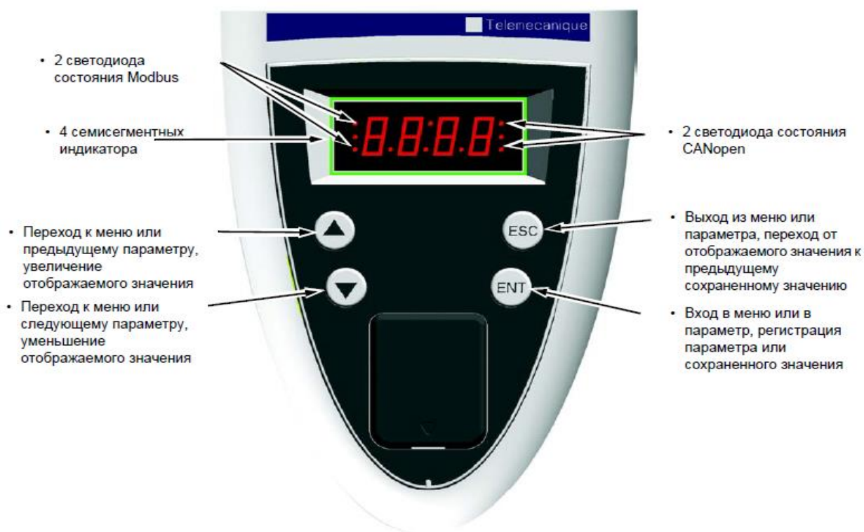
Рисунок 5. Встроенный терминал
