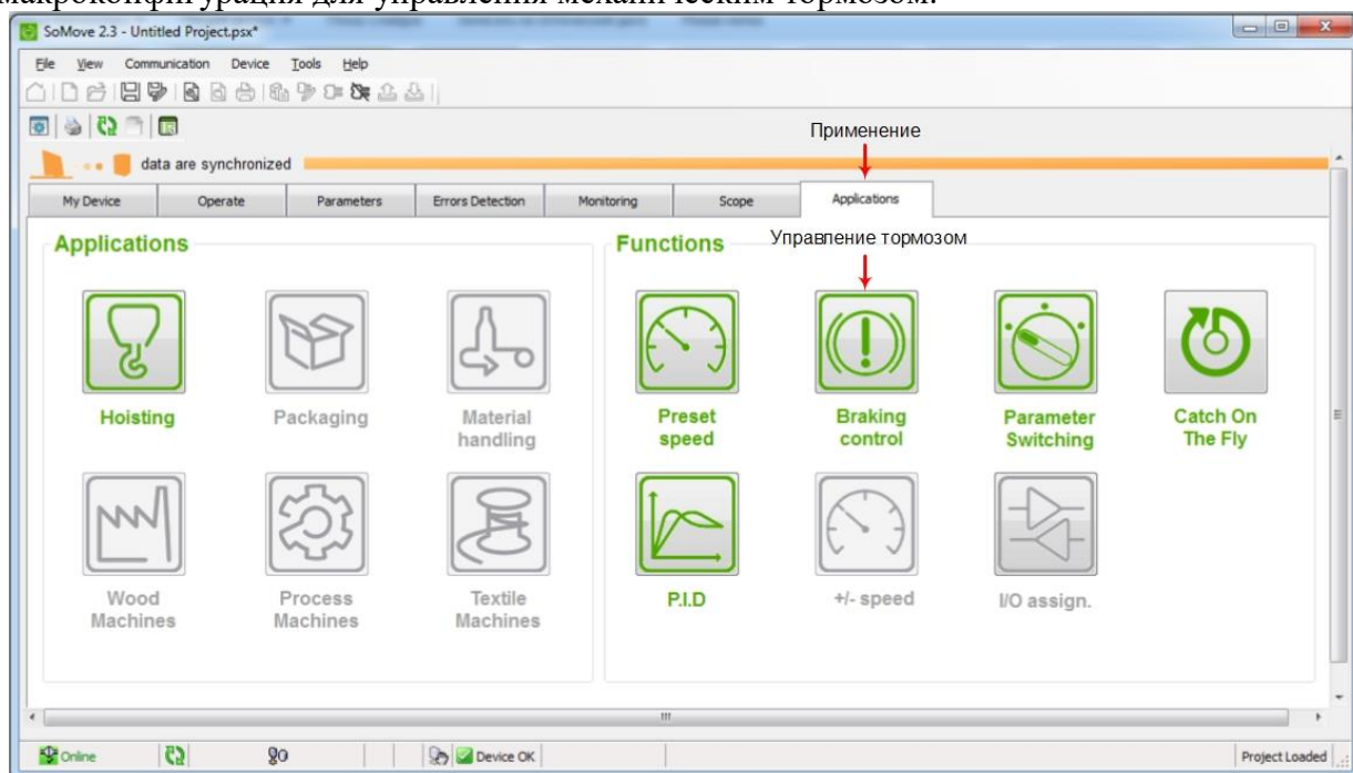
Рисунок 16 – Вкладка «Применение»
