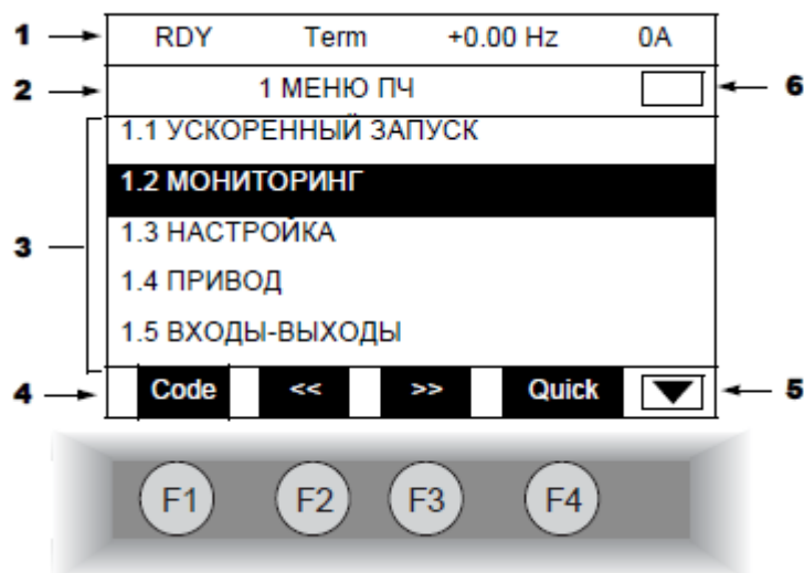
Рисунок 2. Графический дисплей
