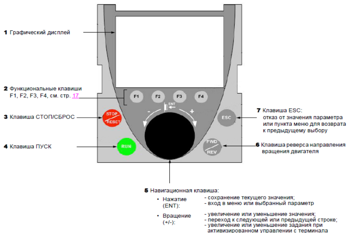
Рисунок 1. Графический терминал
