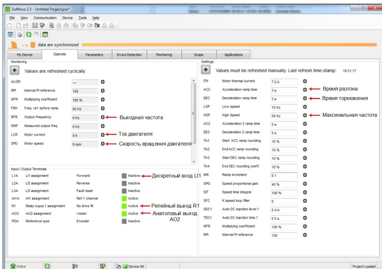
Рисунок 10 – Вкладка управление
