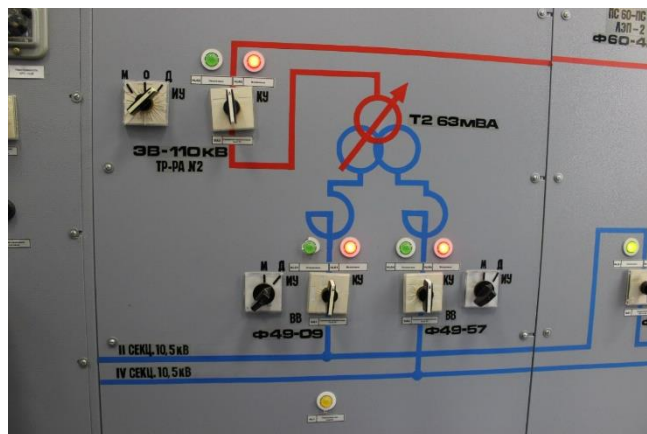
Рис 31 – Мнемосхема
