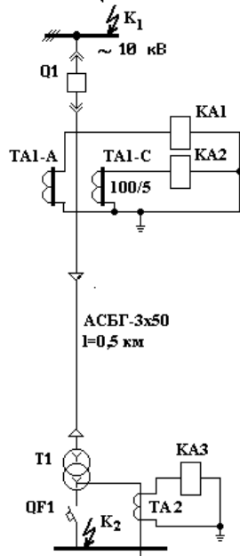
Поясняющая схема
