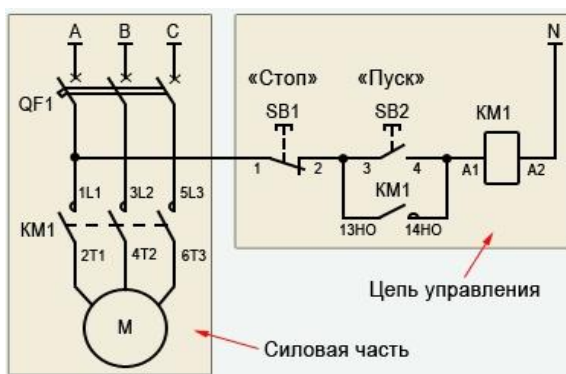
Рис.7 – Обозначения видов цепей на принципиальной схеме
