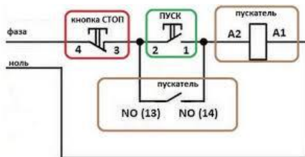
Рис.7 – Обозначения видов цепей на принципиальной схеме
