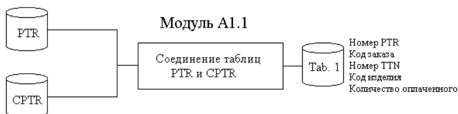
Рис. 5.8. Функционально-технологическая схема модуля A1.1
