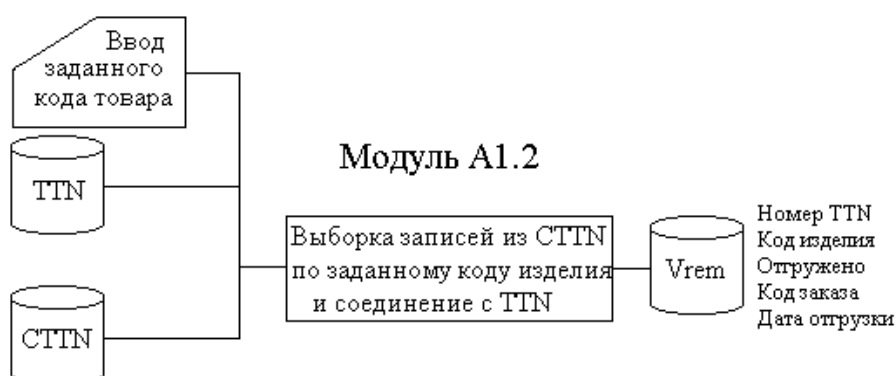
Рис. 5.9. Функционально-технологическая схема модуля A1.2
