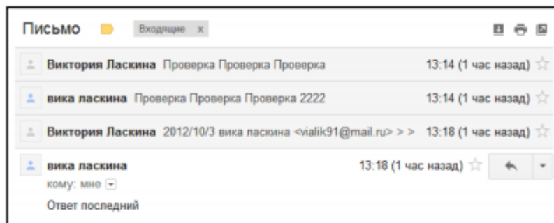
Рисунок 1.17 – Цепочка сообщений
