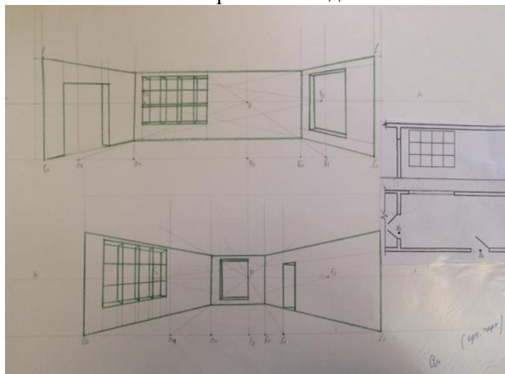
Рис.6. Построение перспективы интерьера методом широкоугольной перспективы
