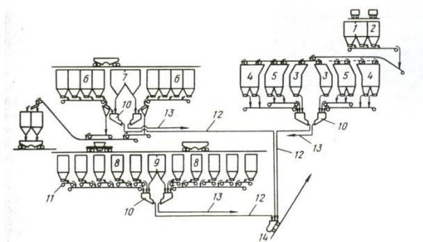
Рис. 6. Схема шихтоподачи доменной печи "Аманды" объемом 2032 м 3 : 1–бункера окатышей; 2,3–бункера известняка; 4–бункера агломерата и руды; 5–бункера окатышей и руды; 6,7–бункера кокша; 8–бункера добавок; 9–бункер скрапа; 10–весовые воронки; 11–13–ленточные весы; 14–скип
