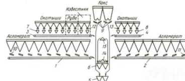
Рис. 4. Система шихтоподачи доменной печи ММК
