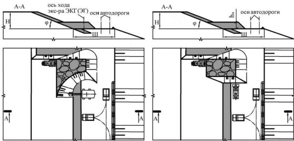
Рис. 6.2 – Разработка двух сближенных пологих пластов ( \phi = 15\text{--}20^\circ ) бульдозерно-рыхлительным агрегатом с погрузкой:
