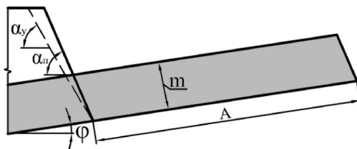
Рис. 3.1 – Параметры заходки по угольному пласту: m – мощность пласта, м; A – ширина заходки, м; \alpha_y ,
