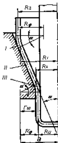
Схема-Схема вытяжки
