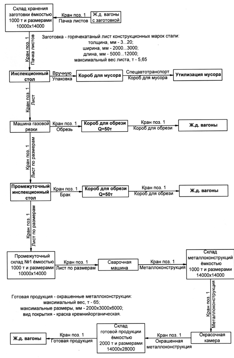
Технологическая схема производства
