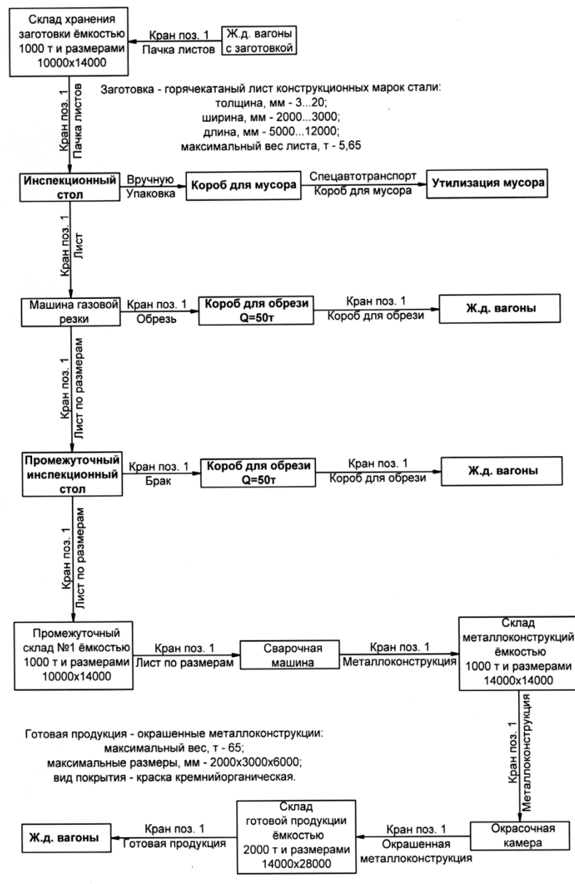
Рисунок 1 - Технологическая схема производства
