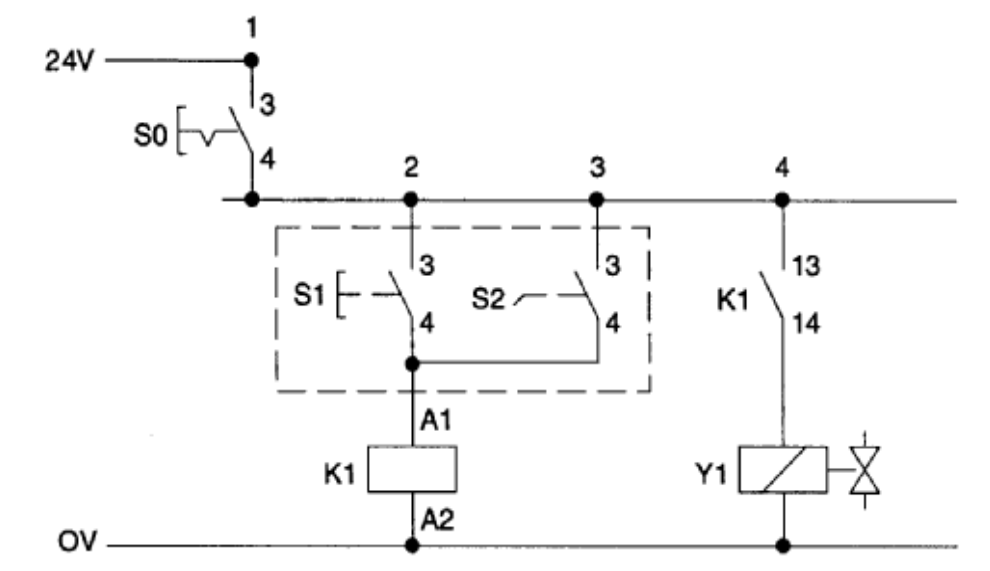
2 электрическая схема
