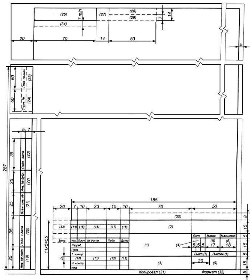
Рис. 3.1. Основная надпись и дополнительные графы для графических документов (чертежей и схем)
