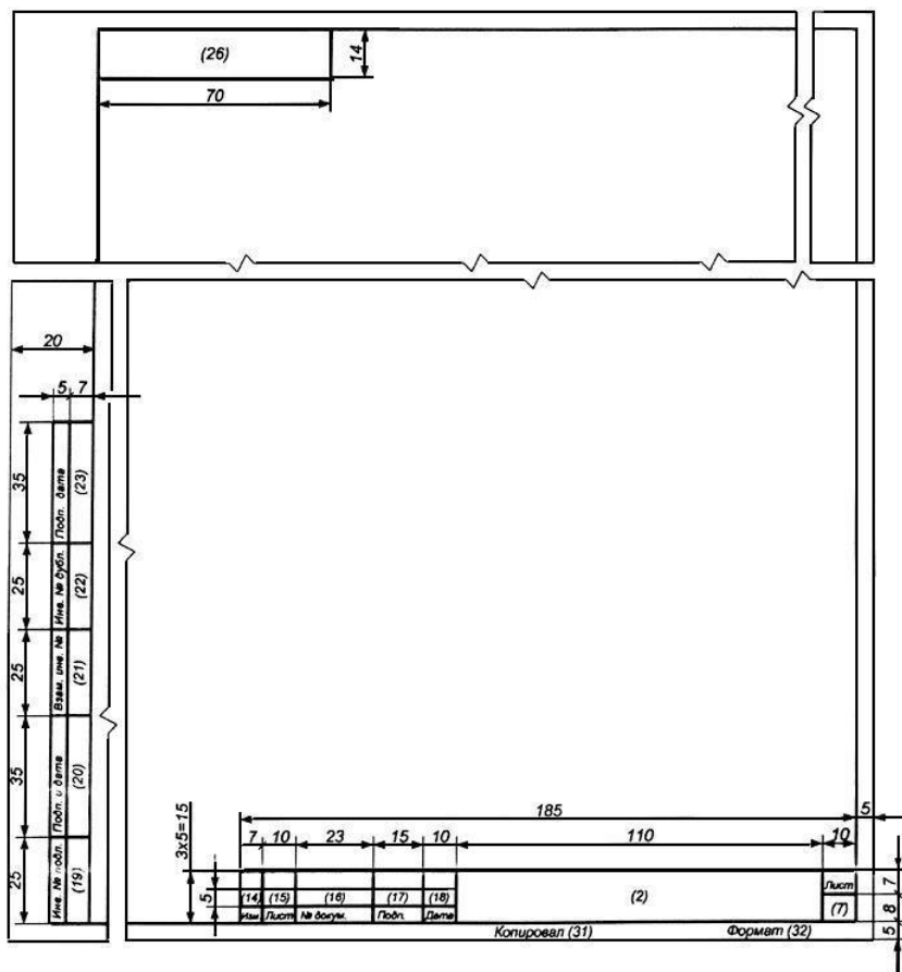
Рис. 3.3. Основная надпись и дополнительные графы для текстовых конструкторских документов (второй и последующие листы)
