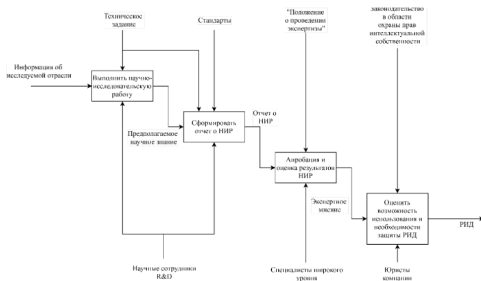
Рисунок - Модель бизнес-процесса «Выполнение научно-исследовательской работы»
