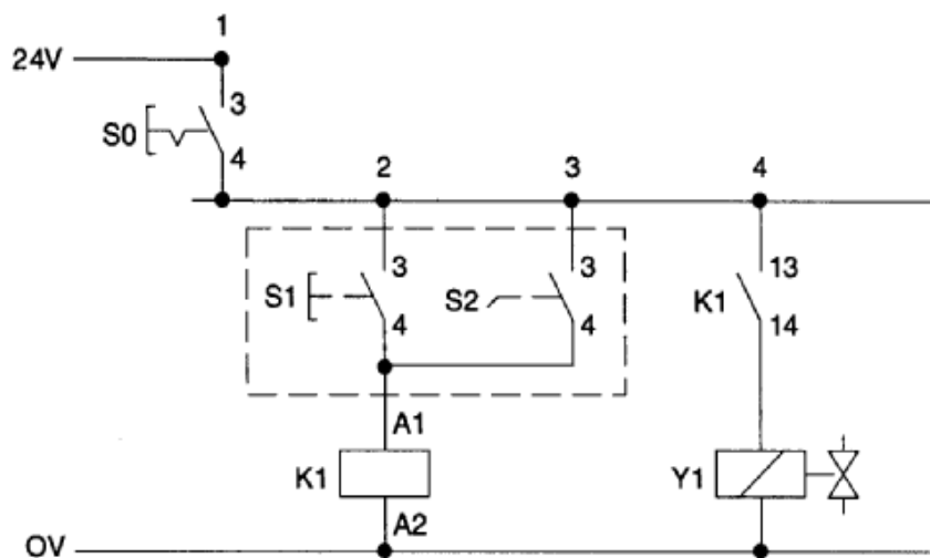
2 электрическая схема
