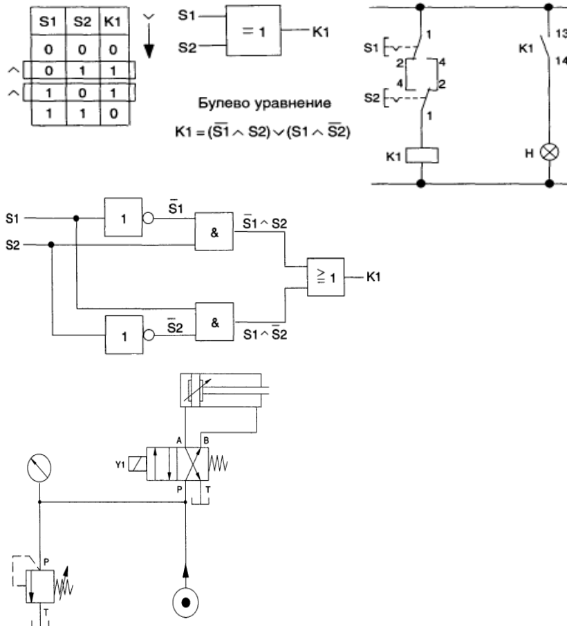
1 электрическая схема с переключающими контактами (самостоятельно)
