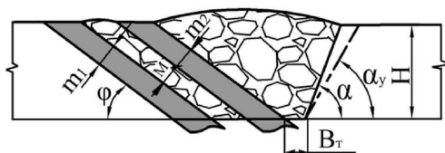
Рис. 5.1 – Параметры залегания пластов на уступе, разрабатываемых по схеме с проходкой разрезной траншеи со стороны кровли верхнего пласта: Н – высота вскрышного уступа, м; \phi – угол залегания пластов, град; m_1 и m_2 – соответственно мощность нижнего и верхнего пласта свиты, м; М – мощность между-пластья, м; B_{т} – ширина разрезной траншеи по дну ( B_{т} = 3\text{ м} ); \alpha_y , \alpha – соответственно устойчивый и рабочий углы откоса вскрышного уступа, град
