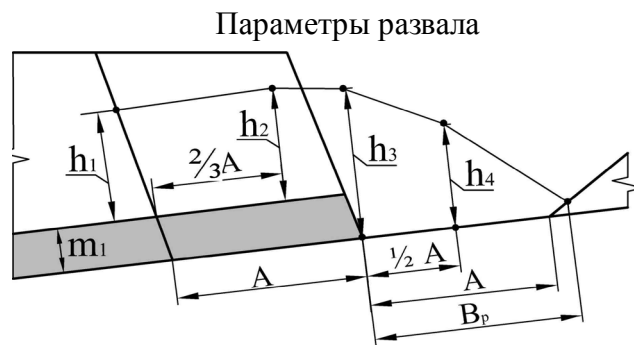
Рис. 2.1 – Параметры начального и конечного статических этапов при построении бестранспортной схемы экскавации:
