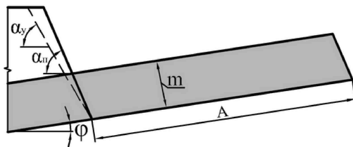
Рис. 3.1 – Параметры заходки по угольному пласту: m – мощность пласта, м; A – ширина заходки, м; α y ,
