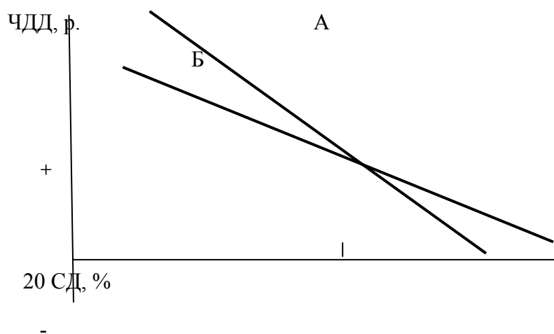
Рис. 2. Определение точки Фишера
