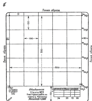
Рисунок 1. Разгафка и номенклатура планшетов масштаба 1:5000 - 1:500 (а) и внешнее оформление планшетов (б)
