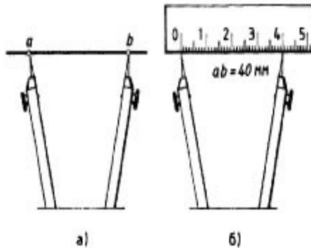
Рисунок 9.10. Циркуль - измеритель
