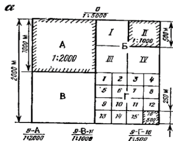
Рисунок 1. Разгафка и номенклатура планшетов масштаба 1:5000 - 1:500 (а) и внешнее оформление планшетов (б)
