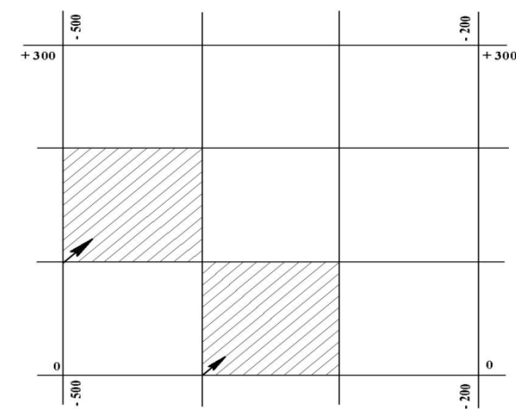
Рис. 7. Оцифровка линий координатной сетки
