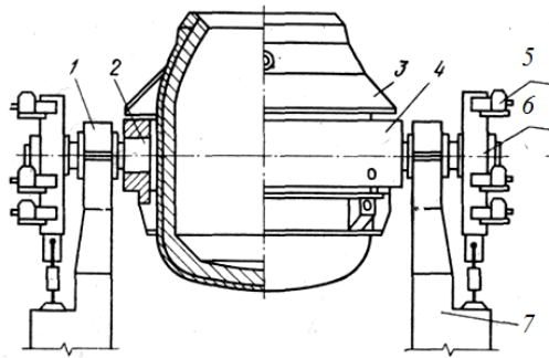
Кислородный конвертер:
