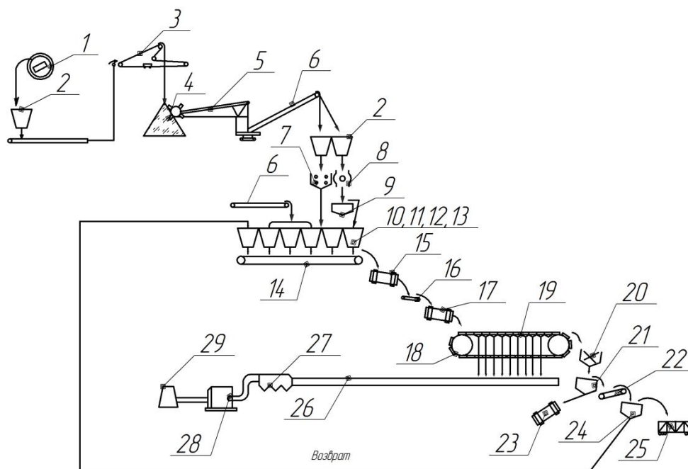
1 - вагоноопрокидыватель; 2 - приемные бункера; 3 - штабелеукладчик; 4 - штабель; 5 - роторный экскаватор; 6 - конвейер; 7-четырёхвалковая дробилка; 8-молотковая дробилка; 9-грохот; 10, 11, 12, 13-бункера соответственно для известняка, кокса, железорудного концентрата и руды, возврата; 14 - смесительный конвейер; 15 - барабанный смеситель; 16 – ленточный транспортер; 17-барабанный окомкователь; 18-агломерационная машина; 19-вакуум-камеры; 20-дробилка, 21, 24 - грохот; 22 - прямолинейный охладитель агломерата; 23 - барабанный охладитель возврата; 25 - агловоз; 26 - газовый коллектор; 27 - пылеочистка; 28 - эксгаустер; 29 - дымовая труба
