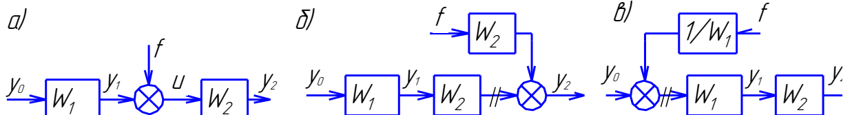
Рис. 5. Схемы переноса сумматора
