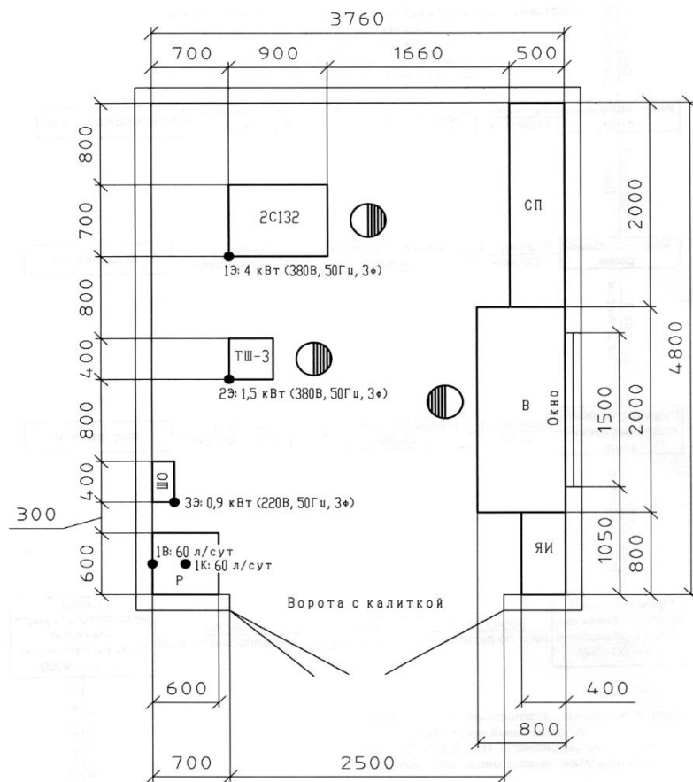
Рисунок 6.3 – Компоновка мастерской
