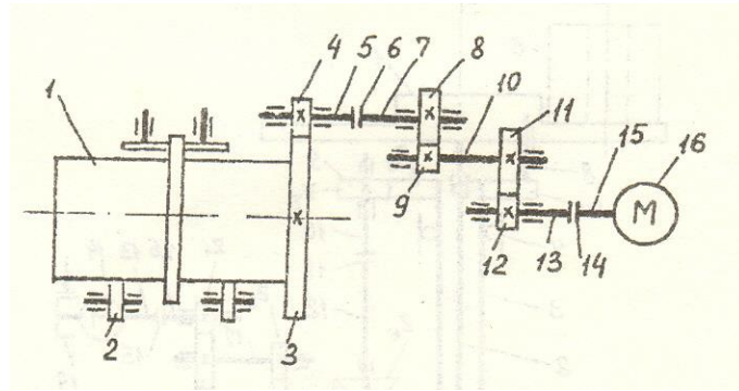
Рис.15. Привод барабанного смесителя-окомкователя
