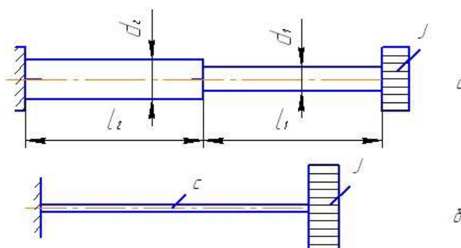
Рис. 7. Расчетная и эквивалентная схемы
