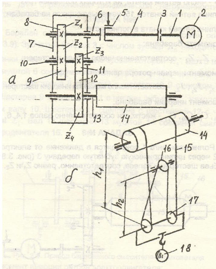
Рис.13. Механизм подъема груза мостового электрического крана: а – кинематическая схема привода;
