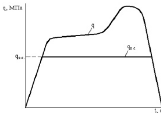
Рис. 1, а. Контроль усилия затяжки колонн в поперечинах: а – состояния стыка между гайкой и поперечиной: q – давление в главных цилиндрах; q_{р.с.} – давление, при котором раскрывается стык
