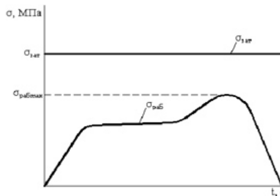
Рис. 1, б. Контроль усилия затяжки колонн в поперечинах: б – контроль запаса по усилию затяжки: \sigma_{зат} – напряжения в колонном стакане поперечины от усилия затяжки; \sigma_{раб.макс} – максимальное напряжение в колонном стакане от рабочей нагрузки; n = \sigma_{зат} / \sigma_{раб.макс} – запас по усилию затяжки
