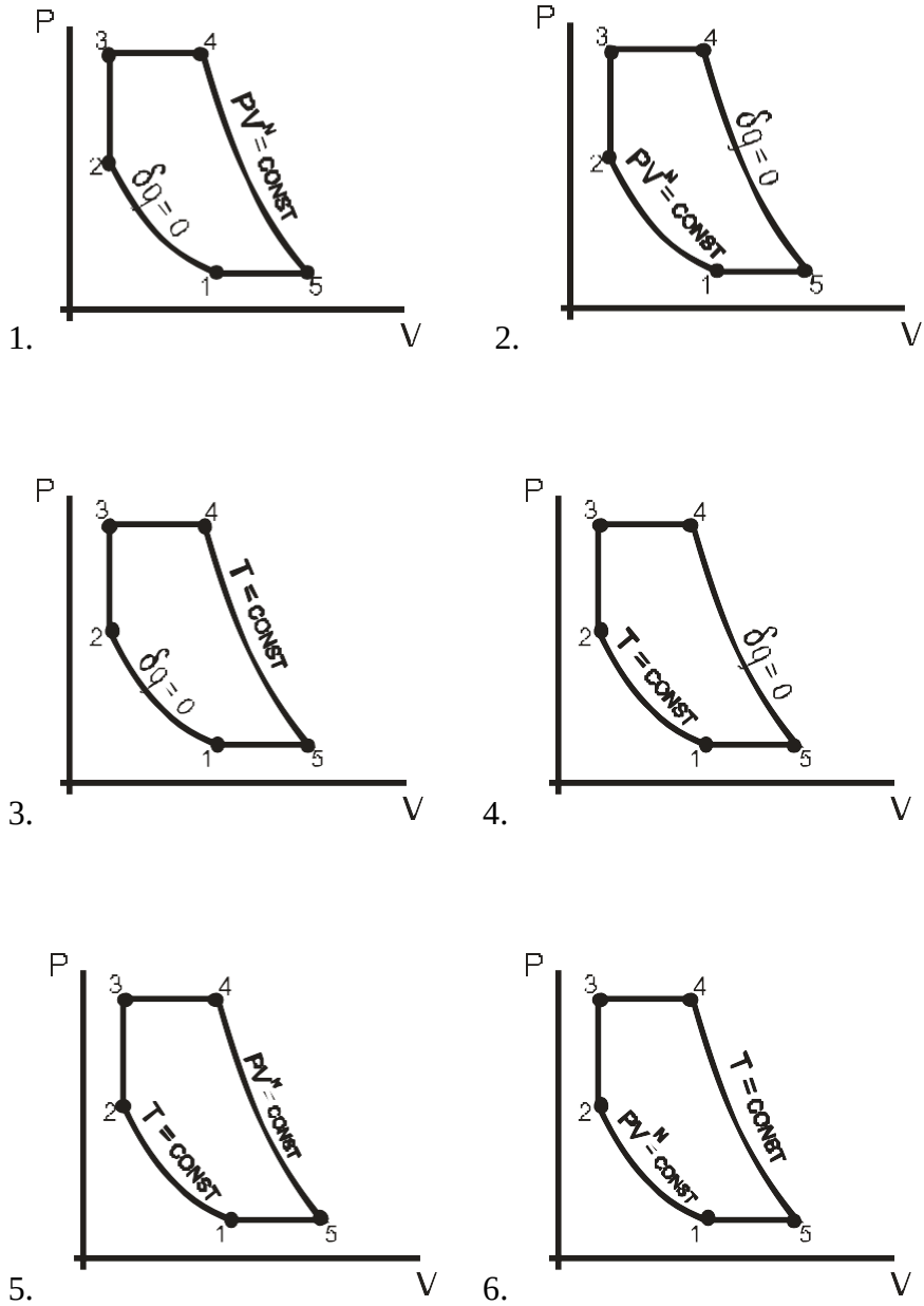
Цикл теплового двигателя (по вариантам):
